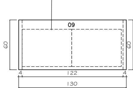
PLANTA MESA ESC. 1/25
