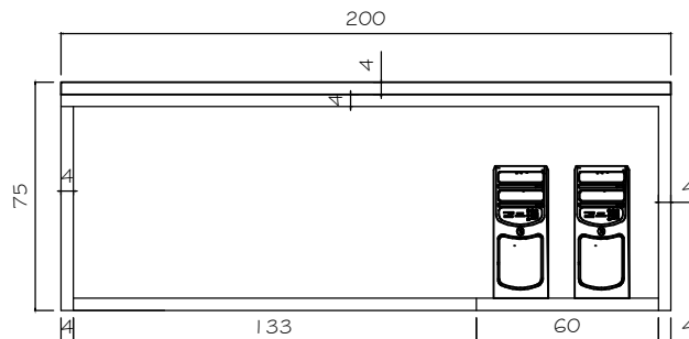
VISTA FRONTAL MESA ESC. 1/25
