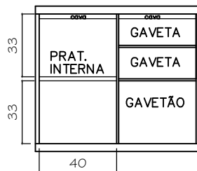
PARTE INTERNA ESC. 1/25
