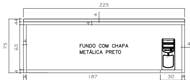
VISTA FRONTAL MESA ESC. 1/25
