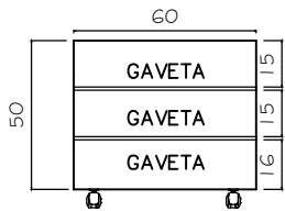
GAVETEIRO FRONTAL ESC. 1/25
