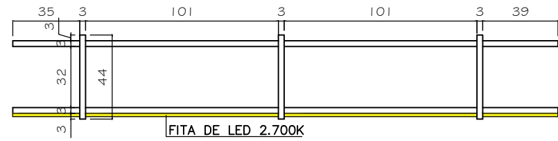
VISTA FRONTAL PRATELEIRA SUSPensa ESC. 1/25
