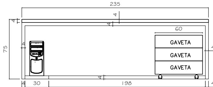
VISTA FRONTAL MESA DE TRABALHO ESC. 1/25
