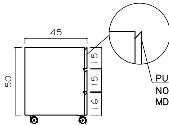
LATERAL GAVETEIRO ESC. 1/25
