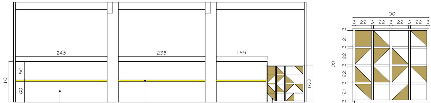
VISTA A ESC. 1/50
