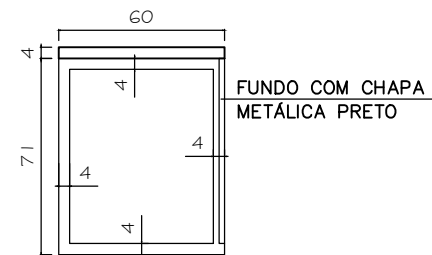
LATERAL DA MESA ESC. 1/25
