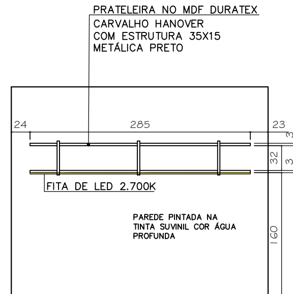
VISTA C ESC. 1/50
