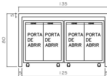
VISTA FRONTAL APARADOR ESC. 1/25
