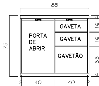
VISTA FRONTAL ARMÁRIO ESC. 1/25
