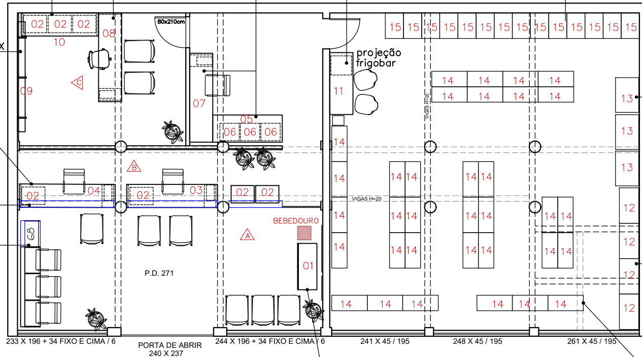
PLANTA DE LAYOUT ESPECIFICAÇÕES ESC. 1/100
