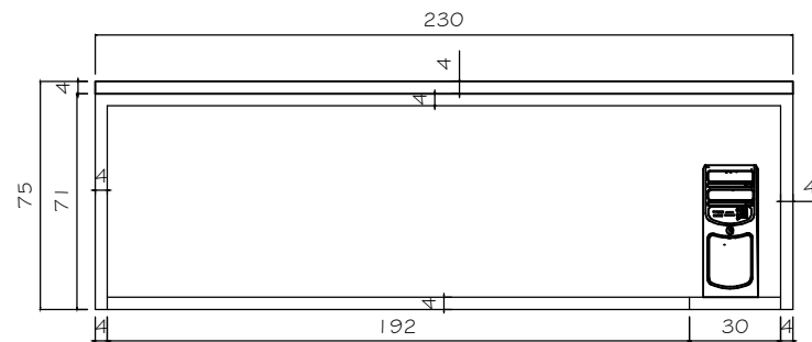
PLANTA MESA DE TRABALHO ESC. 1/25
