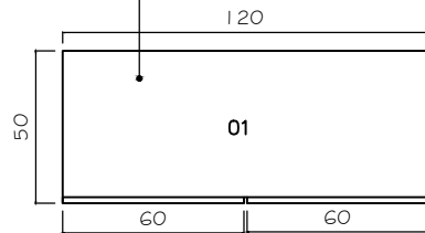
PLANTA MESA DO CAFÉ ESC. 1/25
