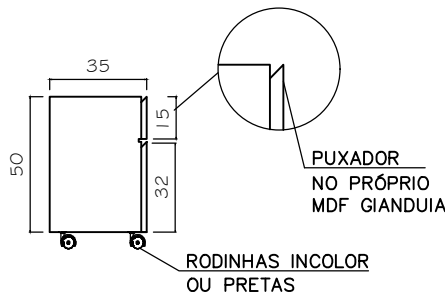
LATERAL GAVETEIRO ESC. 1/25
