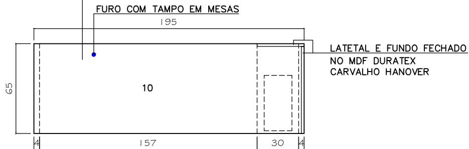
PLANTA MESA ESC. 1/25
