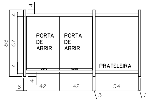
VISTA FRONTAL ARMÁRIO SUSPENSO ESC. 1/25
