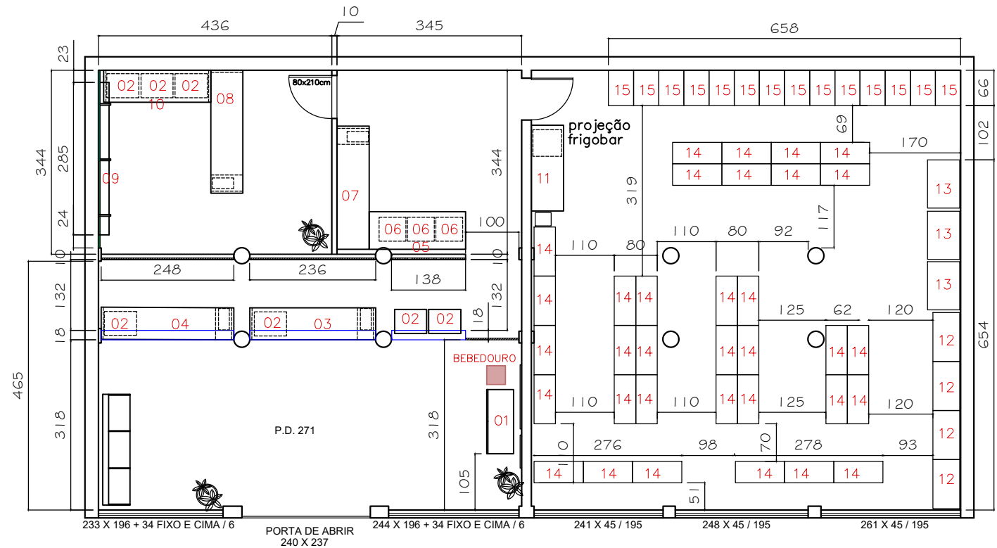
PLANTA DE LAYOUT COM MEDIDAS GERAIS ESC. 1/100
