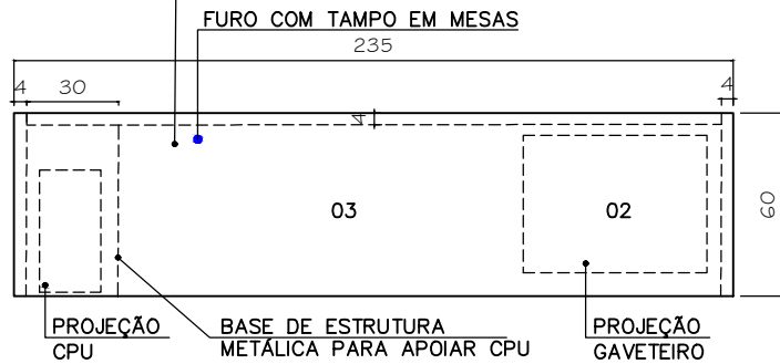
PLANTA MESA DE TRABALHO ESC. 1/25
