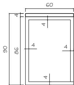
LATERAL DA MESA ESC. 1/25
