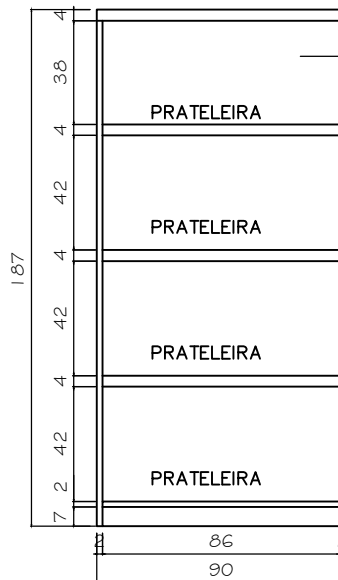
FRENTE ESTANTE ESC. 1/25
