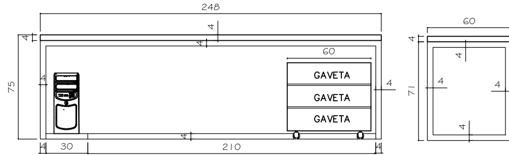
VISTA FRONTAL MESA DE TRABALHO ESC. 1/25
