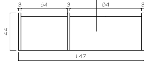
PLANTA ARMÁRIO SUSPENSO ESC. 1/25
