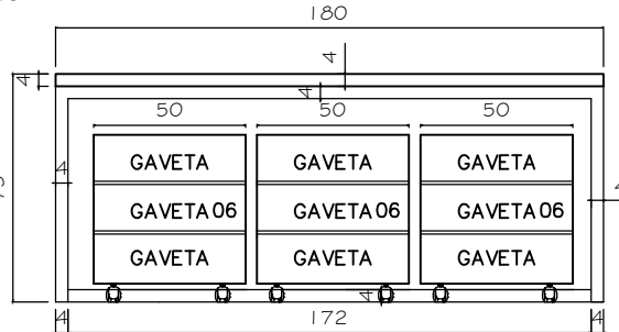
VISTA FRONTAL MESA DE TRABALHO ESC. 1/25
