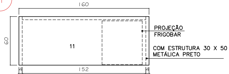
PLANTA MESA DE CAFÉ E ÁGUA ESC. 1/25
