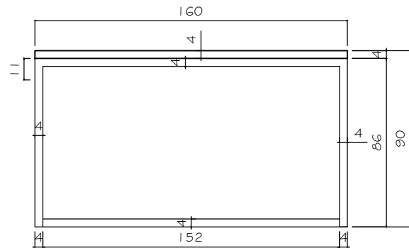
VISTA FRONTAL MESA ESC. 1/25
