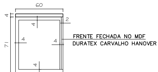
LATERAL DA MESA ESC. 1/25
