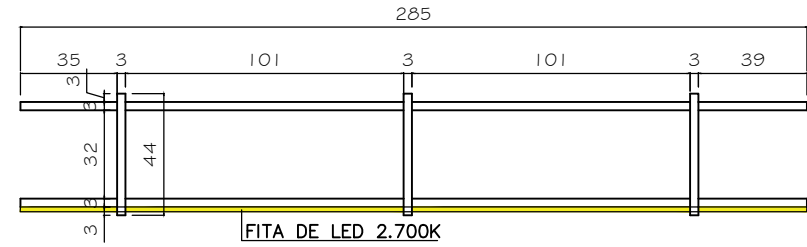
VISTA FRONTAL PRATELEIRA SUSPENSA ESC. 1/25
