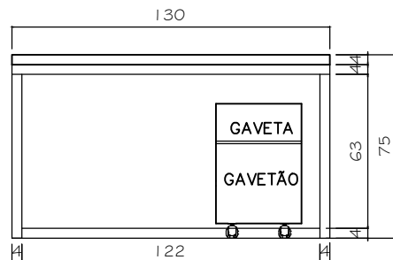
VISTA FRONTAL MESA ESC. 1/25
