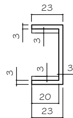
LATERAL PRATELEIRAS ESC. 1/25
