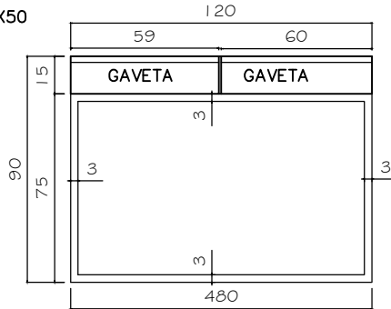
MESA FRONTAL ESC. 1/25
