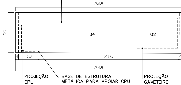
PLANTA MESA DE TRABALHO ESC. 1/25
