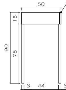
MESA LATERAL ESC. 1/25
