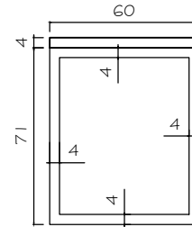
LATERAL DA MESA ESC. 1/25
