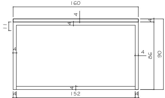
VISTA FRONTAL MESA ESC. 1/25
