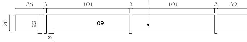
PLANTA PRATELEIRA SUSPENSA ESC. 1/25
