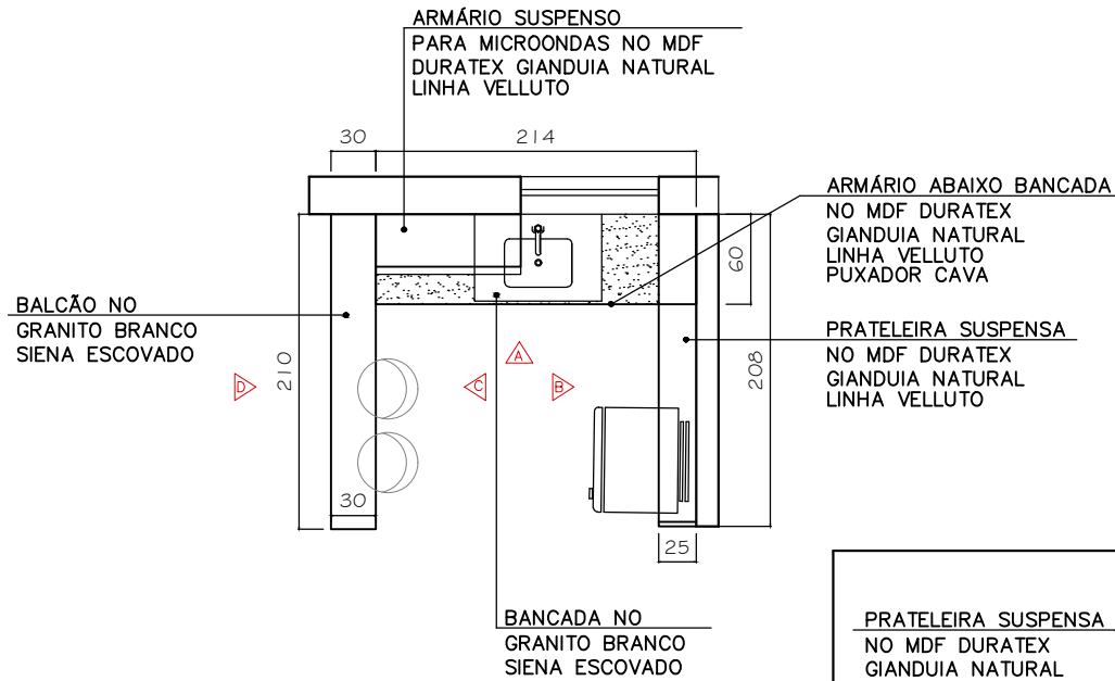
PLANTA COZINHA ESC. 1/50
