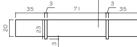
PLANTA PRATELEIRAS ESC. 1/25
