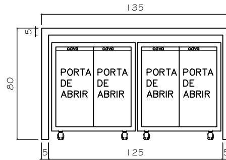
VISTA FRONTAL APARADOR ESC. 1/25
