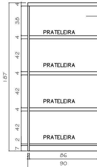
FRENTE ESTANTE ESC. 1/25
