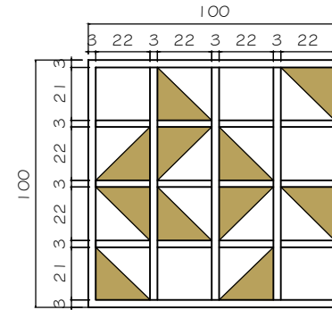
DETALHE DA DIVISÓRIA ESC. 1/25
